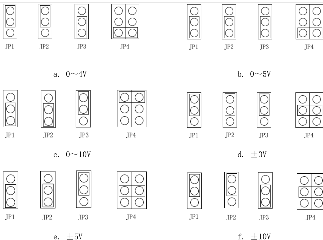
图 2 A / D 量程选择
