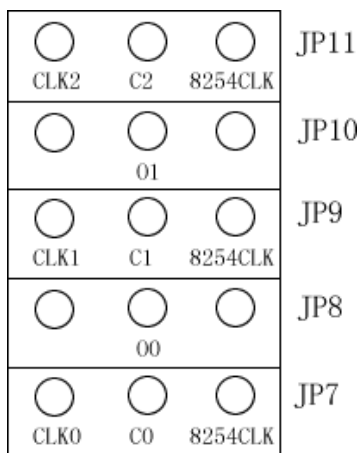
图 4 JP7—JP11 的定义
