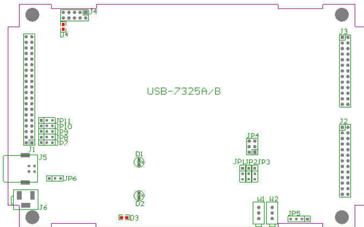
图 1 主要可调整元件位置图
